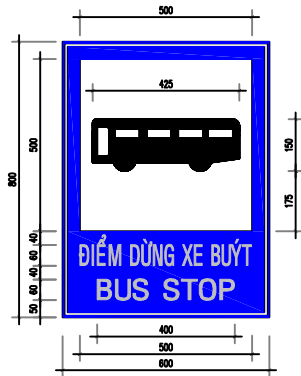
MẪU SỐ 1: BIỂN BÁO "ĐIỂM DỪNG XE BUÝT" ĐƯỜNG ĐÔ THỊ
