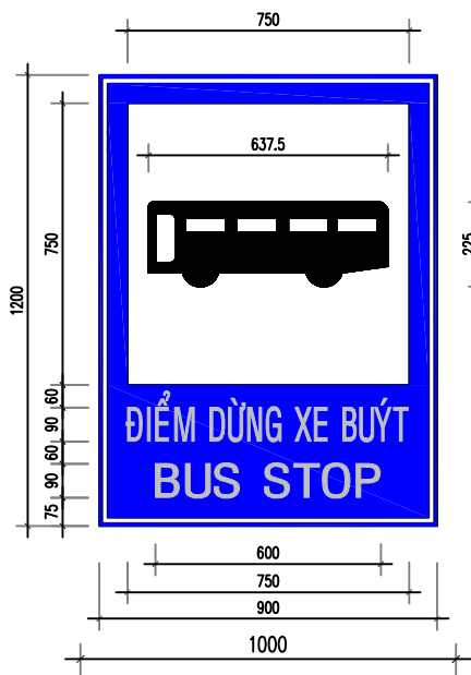
MẪU SỐ 3: BIỂN BÁO "ĐIỂM DỪNG XE BUÝT" ĐƯỜNG ĐÔI NGOÀI ĐÔ THỊ
