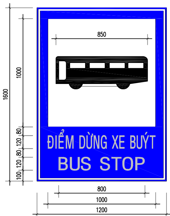
MẪU SỐ 3: BIỂN BÁO "ĐIỂM DỪNG XE BUÝT" ĐƯỜNG ĐÔI NGOÀI ĐÔ THỊ
